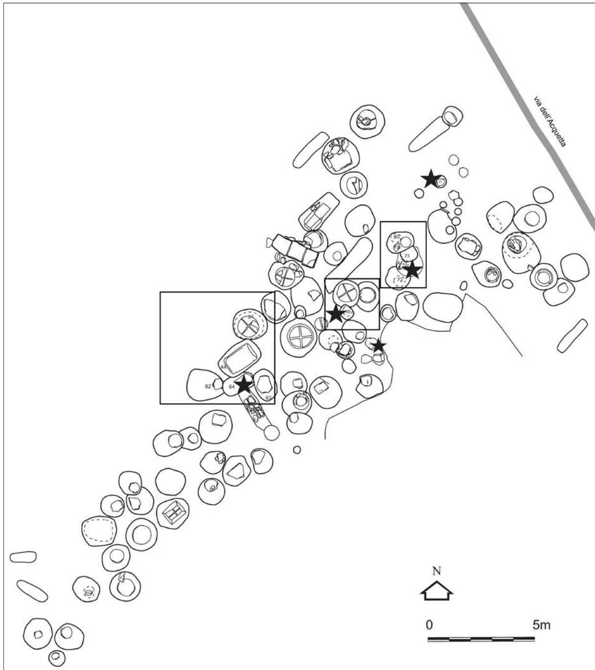
Fig. 16. Planimetria del settore meridionale.
